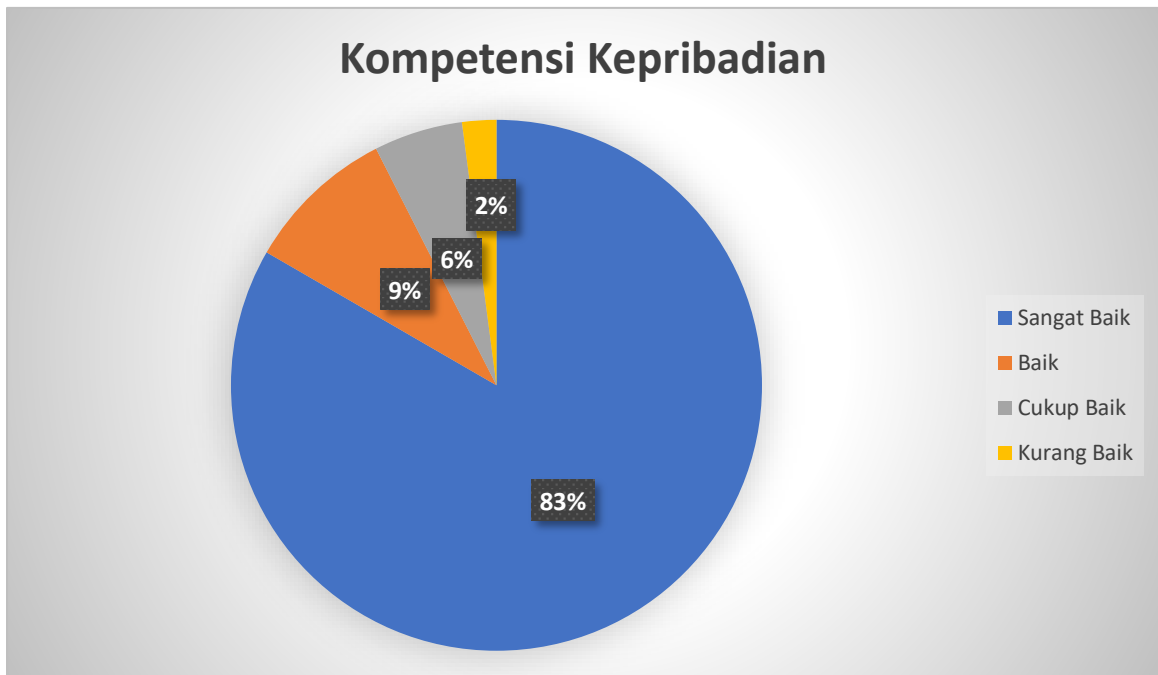
Gambar 3. Kompetensi Kepribadian
