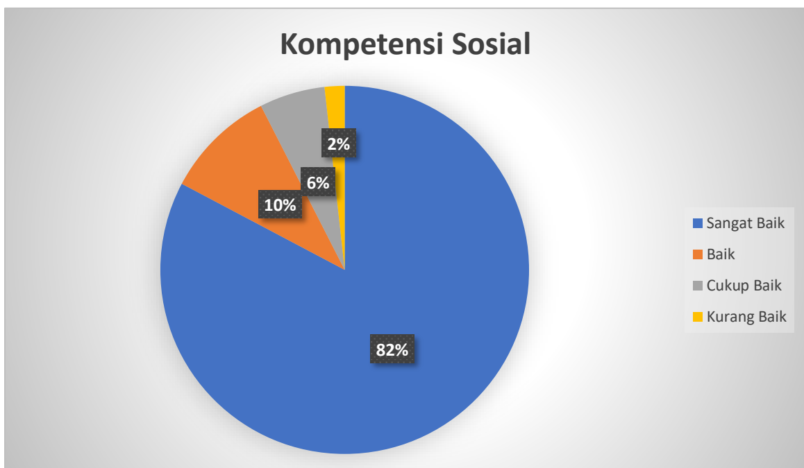
Gambar 4. Kompetensi Sosial
